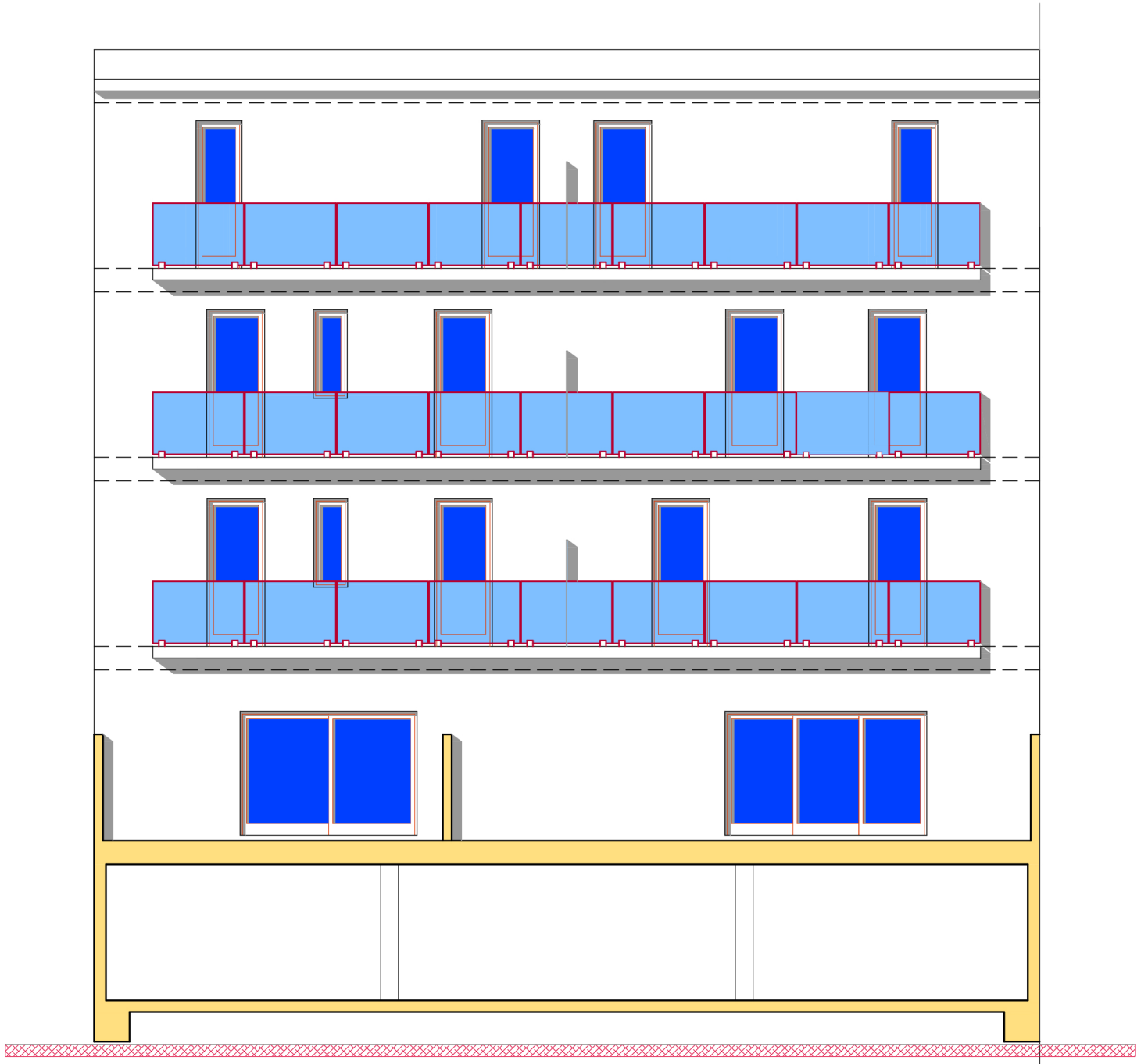
ALZADO POSTERIOR
