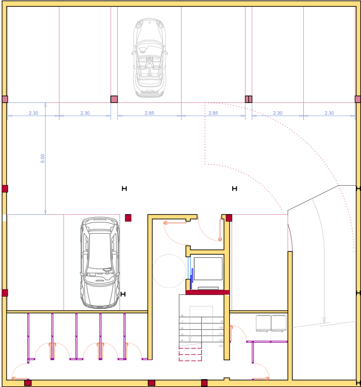
PLANTA SOTANO SUP. CONSTRUIDA 275,62 m 2
